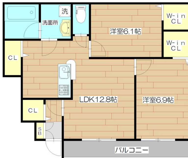
【間取り図】
